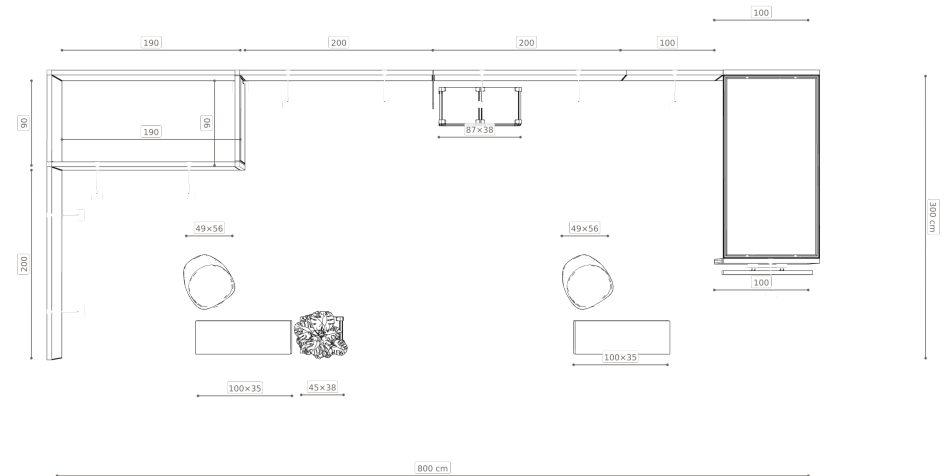
Rzut — szerokości modułów i mebli
