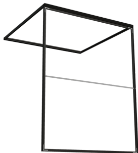
Sufit 200 × 200 cm bez LED ze ścianą frontową 200 × 250 cm 200 × 200 cm
