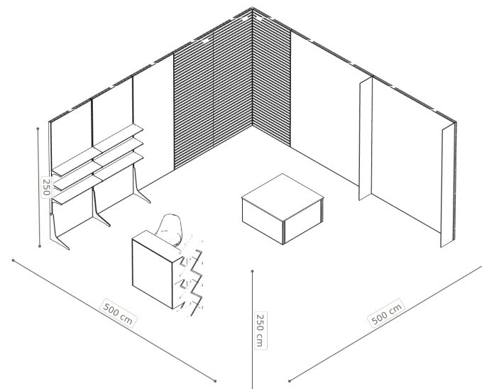
Izometria — wysokości elementów
