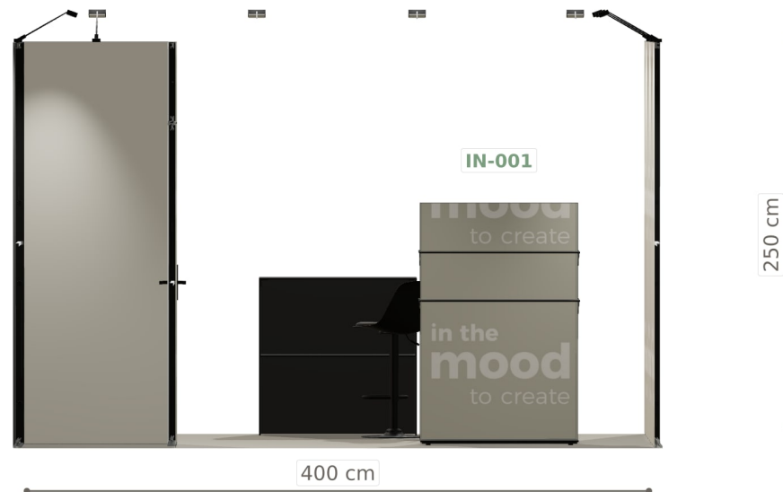
Elewacja od tyłu
