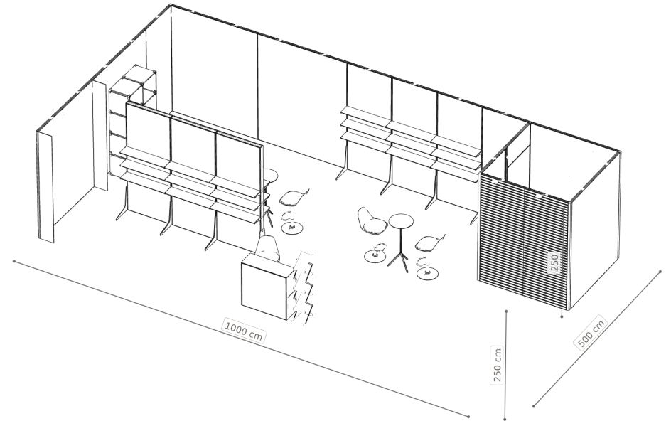
Izometria — wysokości elementów
