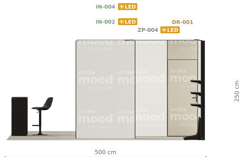
Elewacja z prawej
