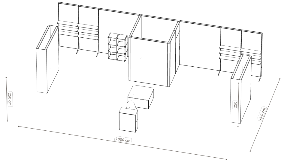
Izometria — wysokości elementów
