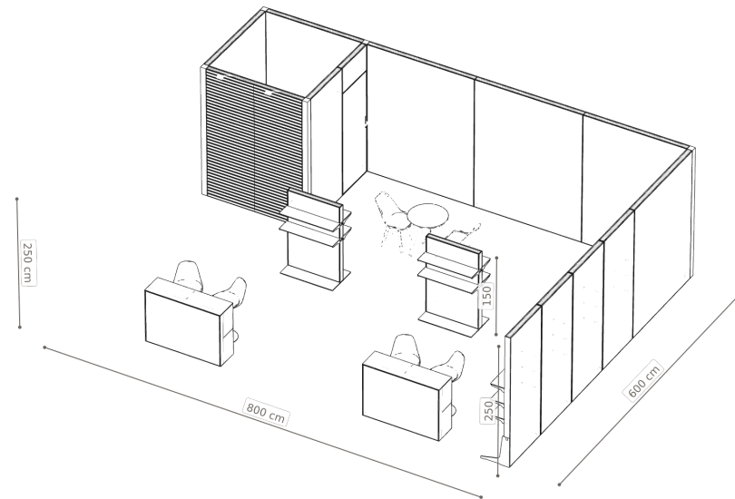
Izometria — wysokości elementów
