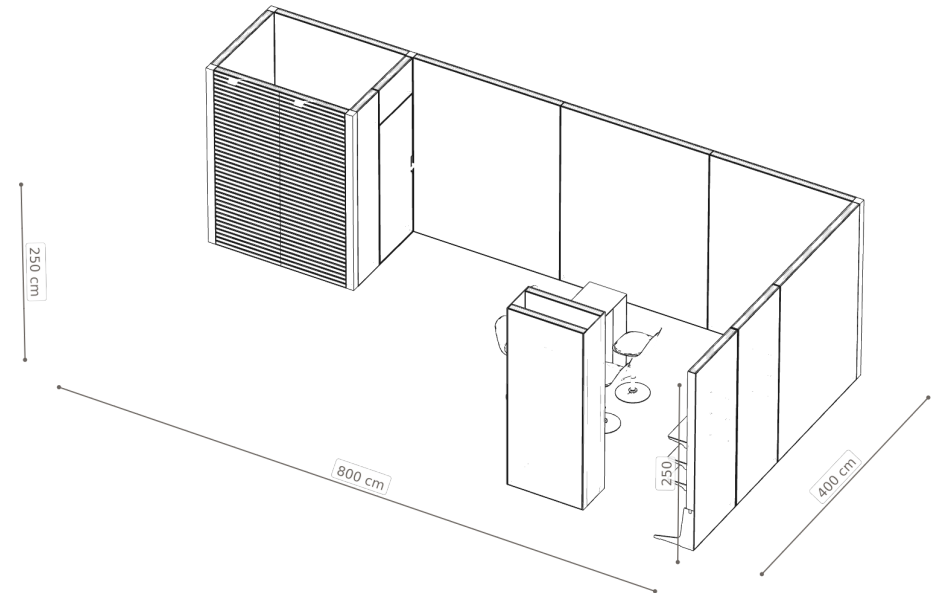
Izometria — wysokości elementów
