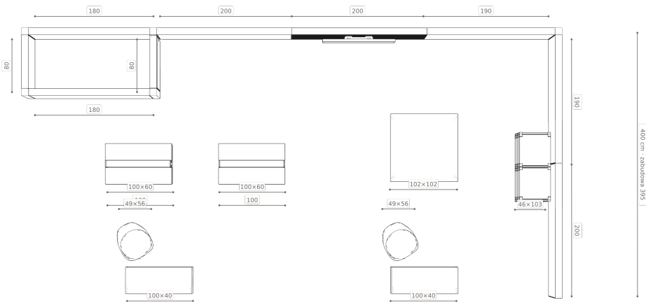
Rzut — szerokości modułów i mebli
