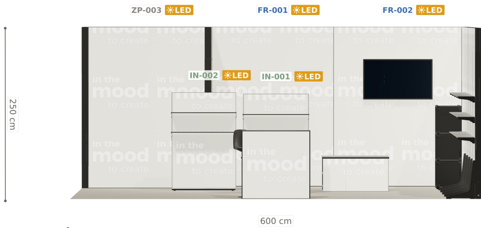
Elewacja ściany tylnej
