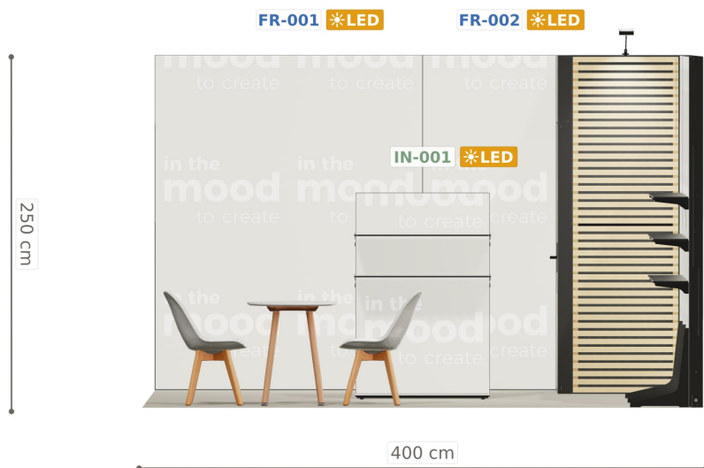
Elewacja ściany tylnej
