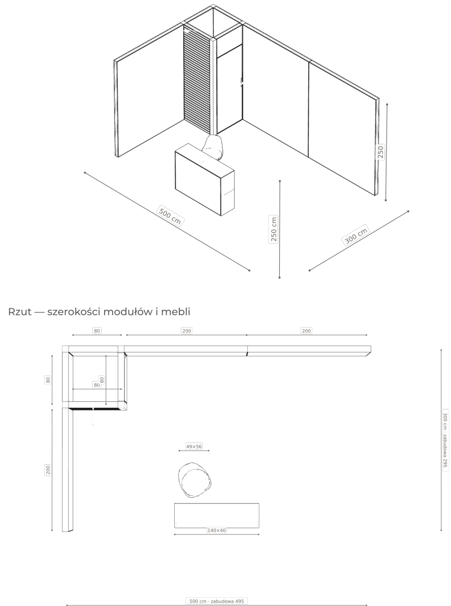
Izometria — wysokości elementów
