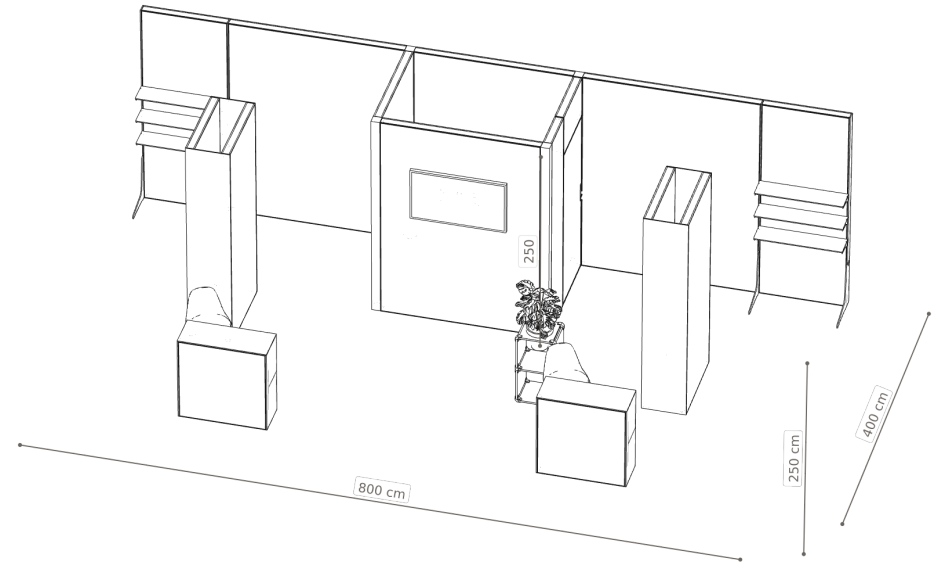
Izometria — wysokości elementów
