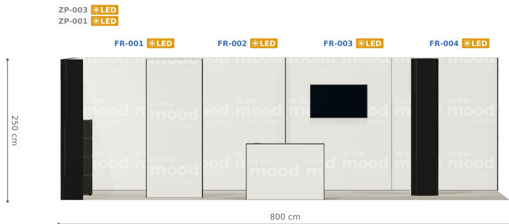
Elewacja ściany tylnej
