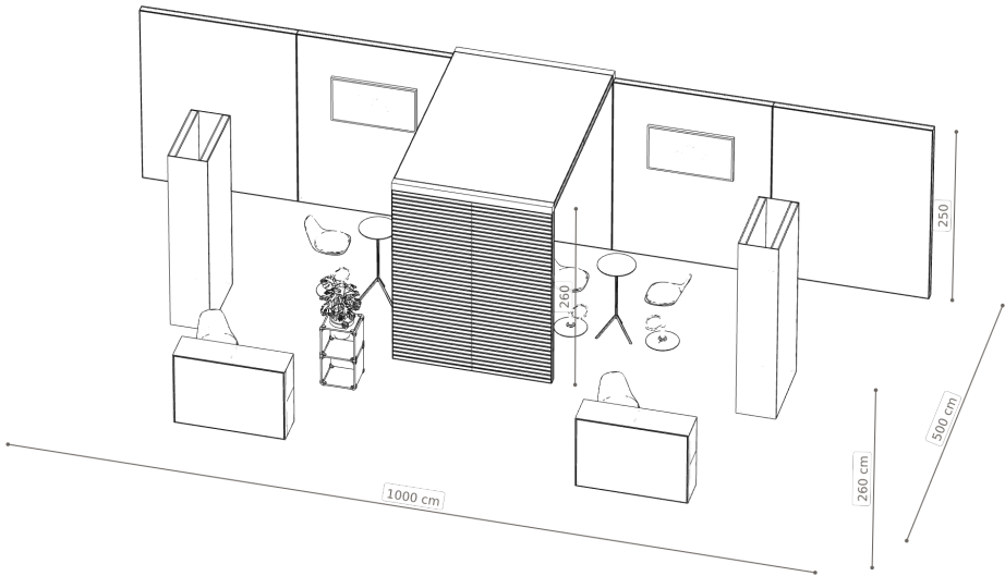
Izometria — wysokości elementów
