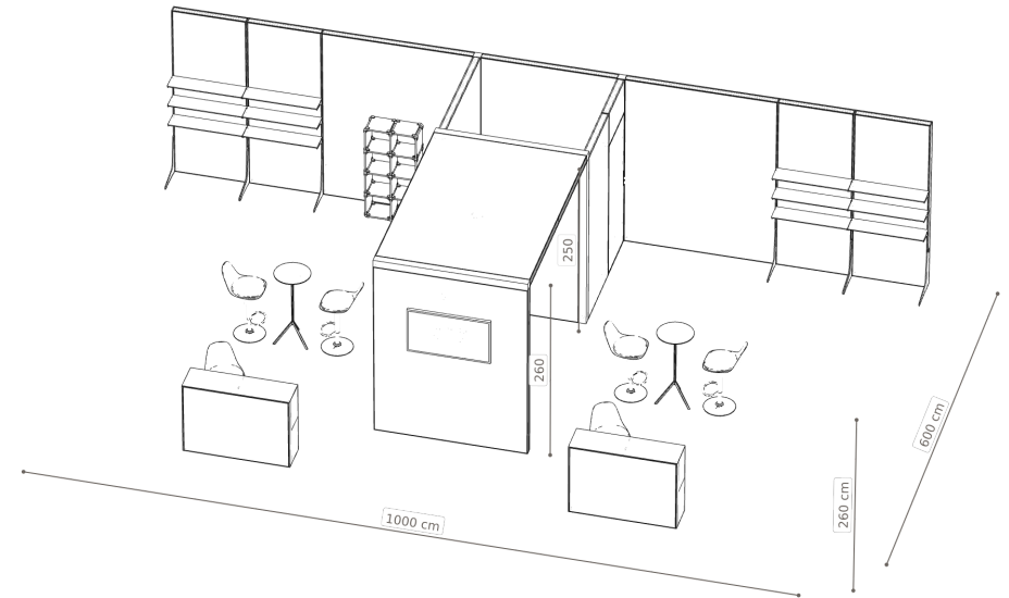
Izometria — wysokości elementów
