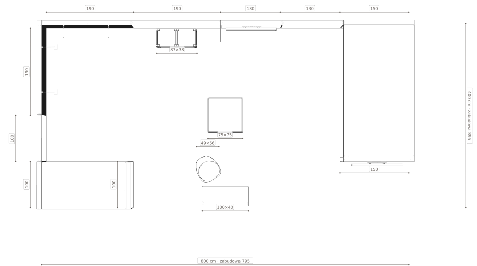
Rzut — szerokości modułów i mebli
