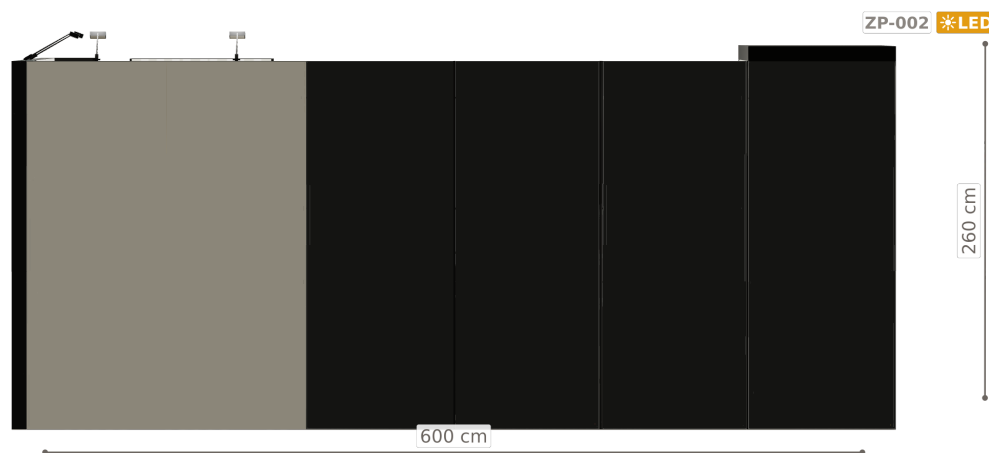
Elewacja od tyłu
