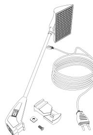
Lampa LED P12 z mocowaniem M100
