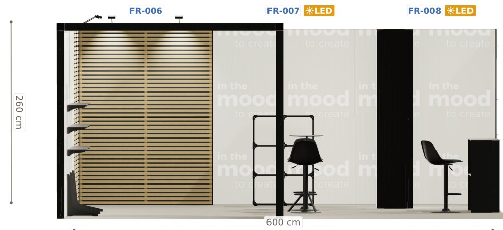
Elewacja ściany prawej
