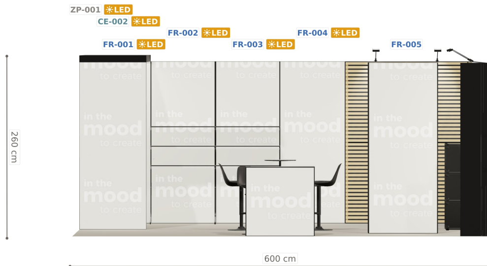
Elewacja ściany tylnej
