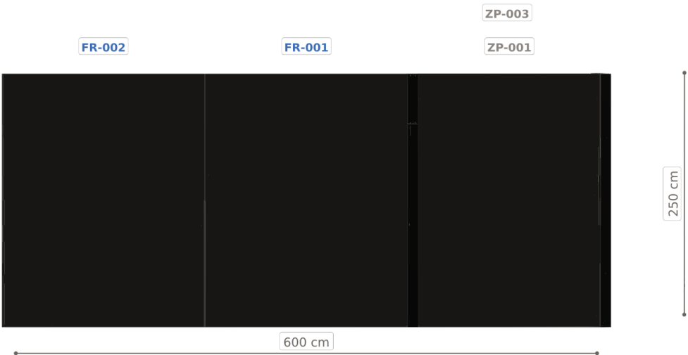
Elewacja tylna
